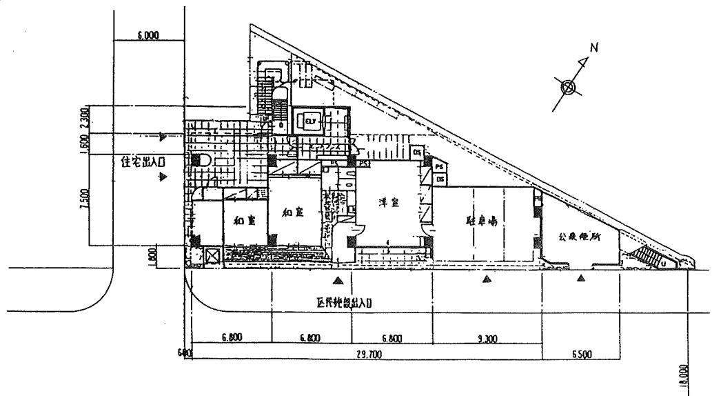
区民館（仮称）1階施設見取図案
